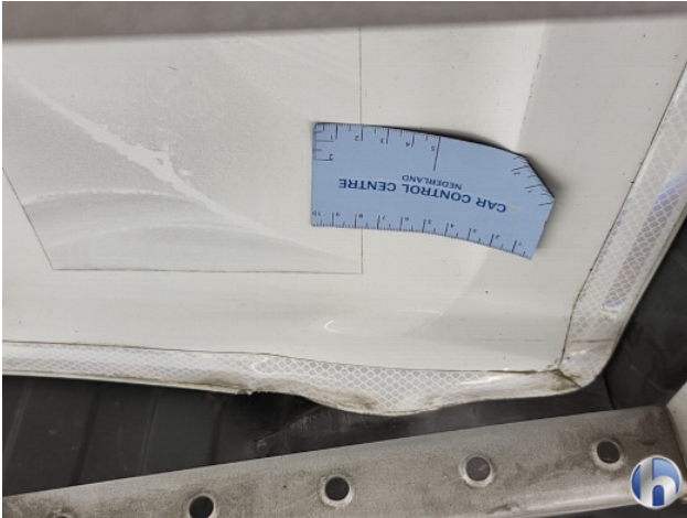
1. Achterbumper Breuk / barst / scheur - Vernieuwen
