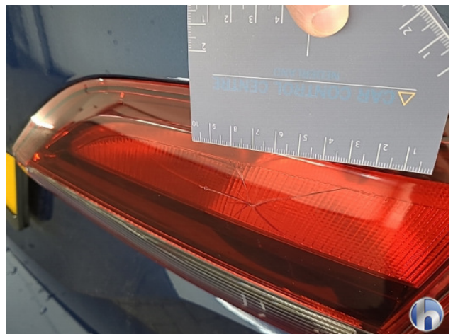
4. Achterlicht rechts Breuk / barst / scheur - Vernieuwen
