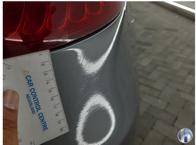
4. Achterlicht rechts Krassen - Vernieuwen
